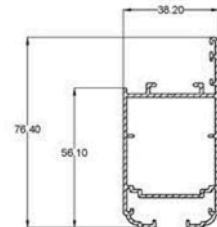
6005 DOOR PANEL
