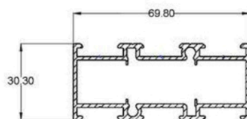
70-01 PERIMETER
