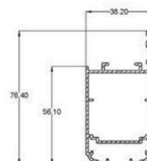
6005 DOOR PANEL
